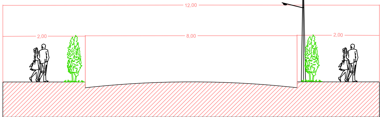
DETALHE TÍPICO DAS ALAMEDAS E RUAS
