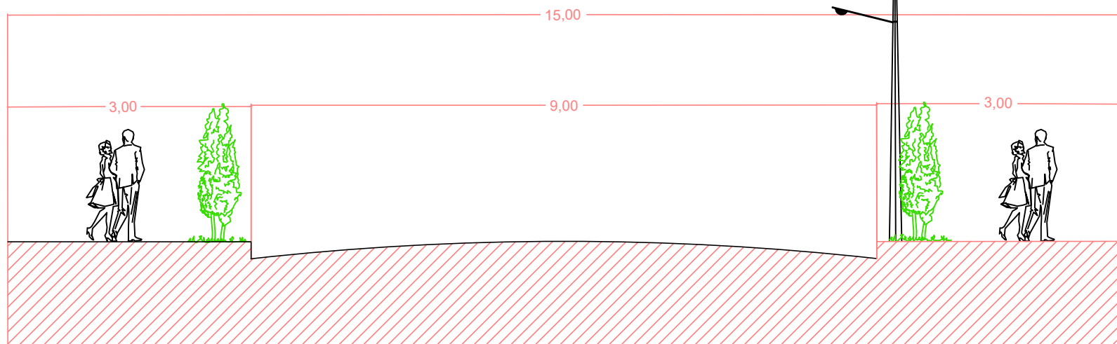
DETALHE TÍPICO DA RUA 5
