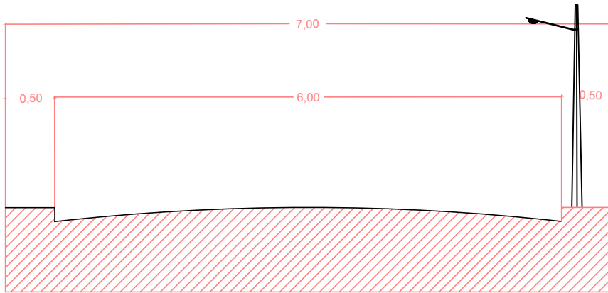
DETALHE TÍPICO DA RUA 12
