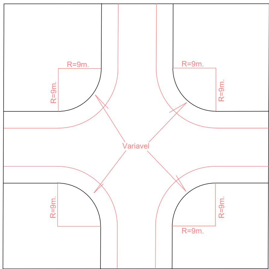
DETALHE DE CONCORDANCIA DAS RUAS E ALAMEDAS
